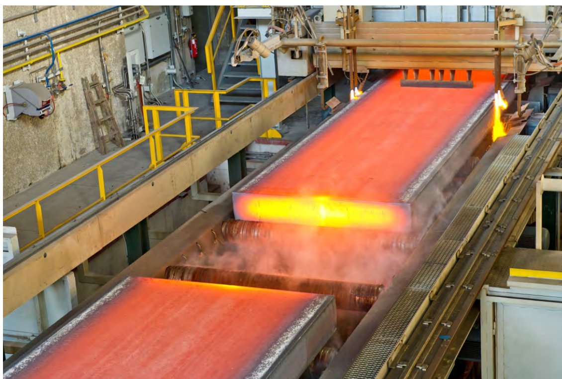
プライメタルズテクノロジーズ製の1ストランド式スラブ連続 casting 機
