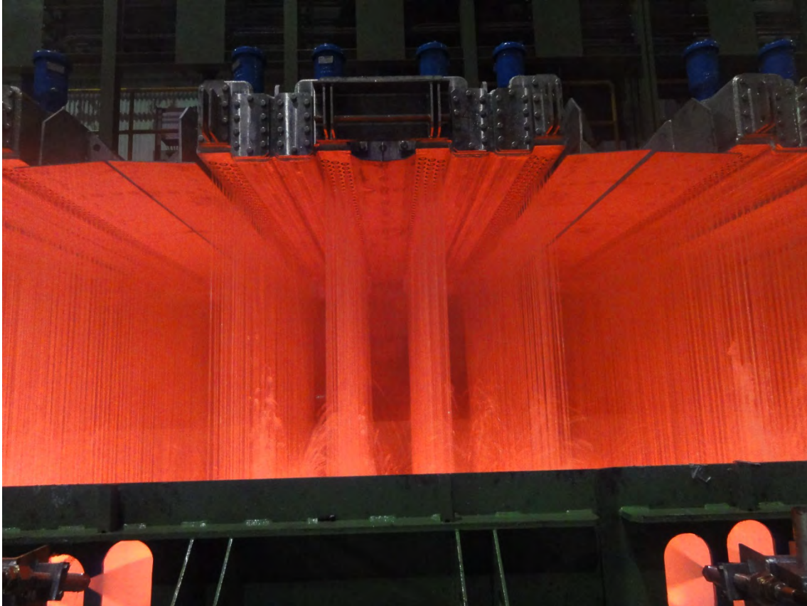
プライメタルズテクノロジーズの熱間圧延機用パワークーリング (写真は画面上部から大量の冷却水が投入されている場面)
